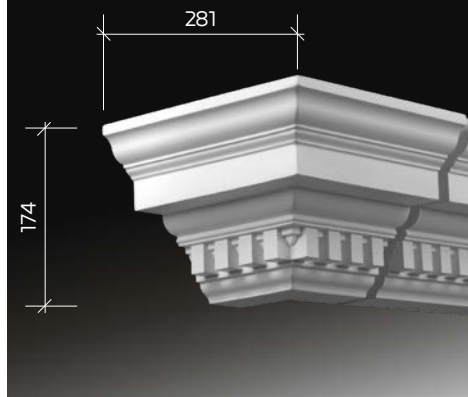
4.32.232 торцевой элемент
