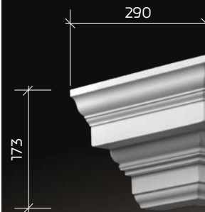
4.32.211 внешний угол
