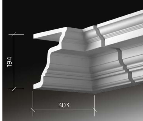
4.38.302 модильон глубина модильона 33 мм
