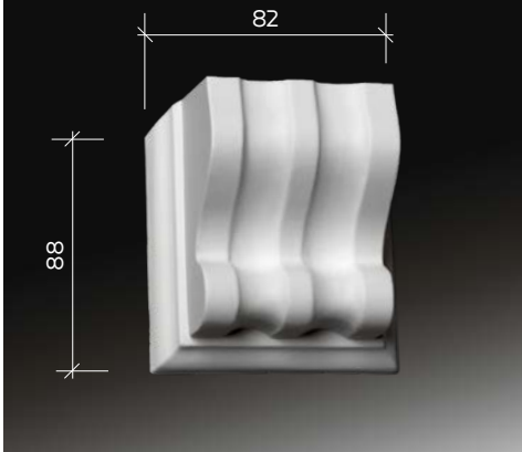
4.08.301 модильон глубина модильона 45 мм
