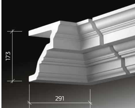
4.32.221 внутренний угол
