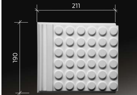
4.05.101 мутул глубина мутула 61 мм
