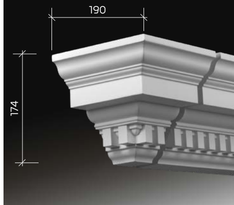
4.32.232 торцевой элемент
