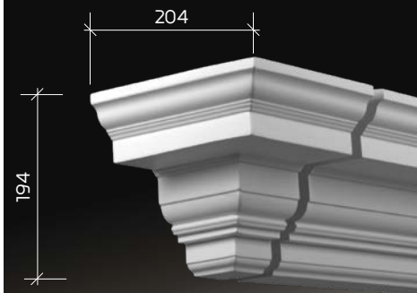
4.32.332 торцевой элемент
