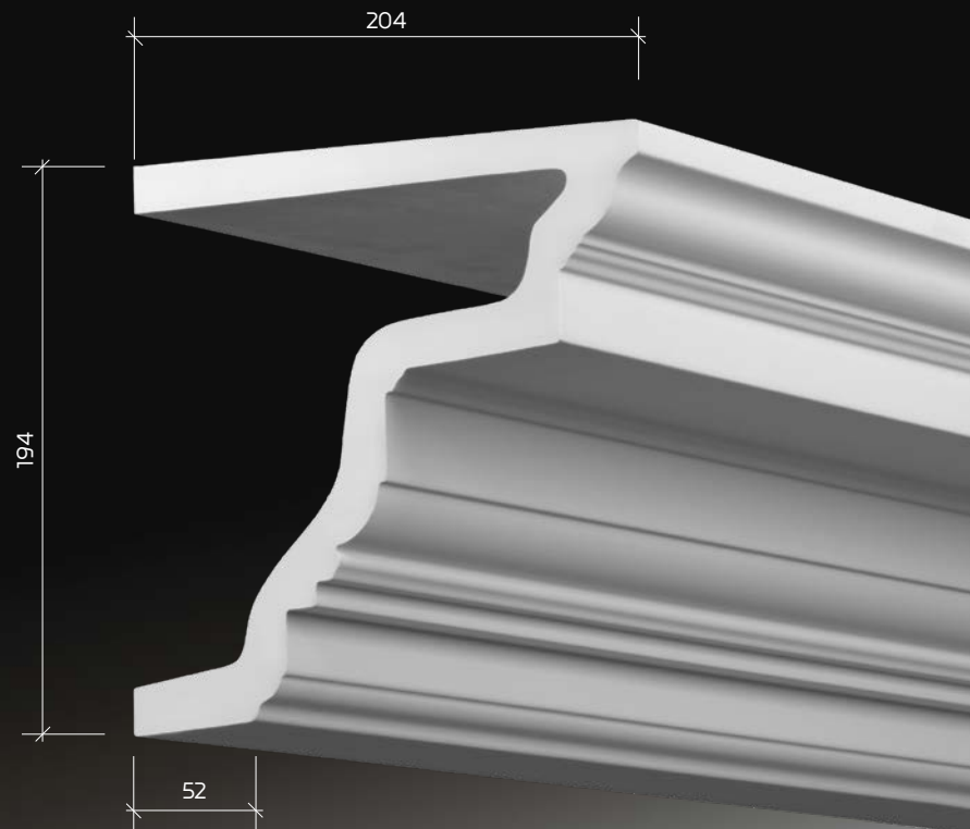
4.32.302 карниз
