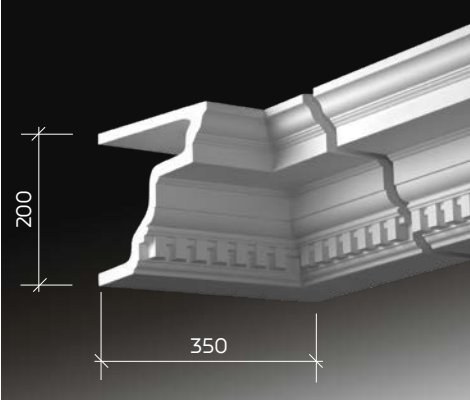
4.08.301 модильон глубина модильона 33 мм
