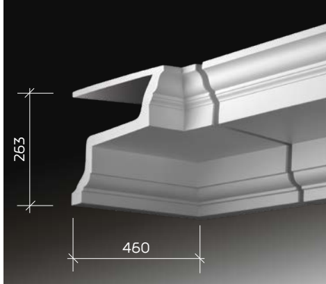
4.05.101 мутул глубина мутула 61 мм
