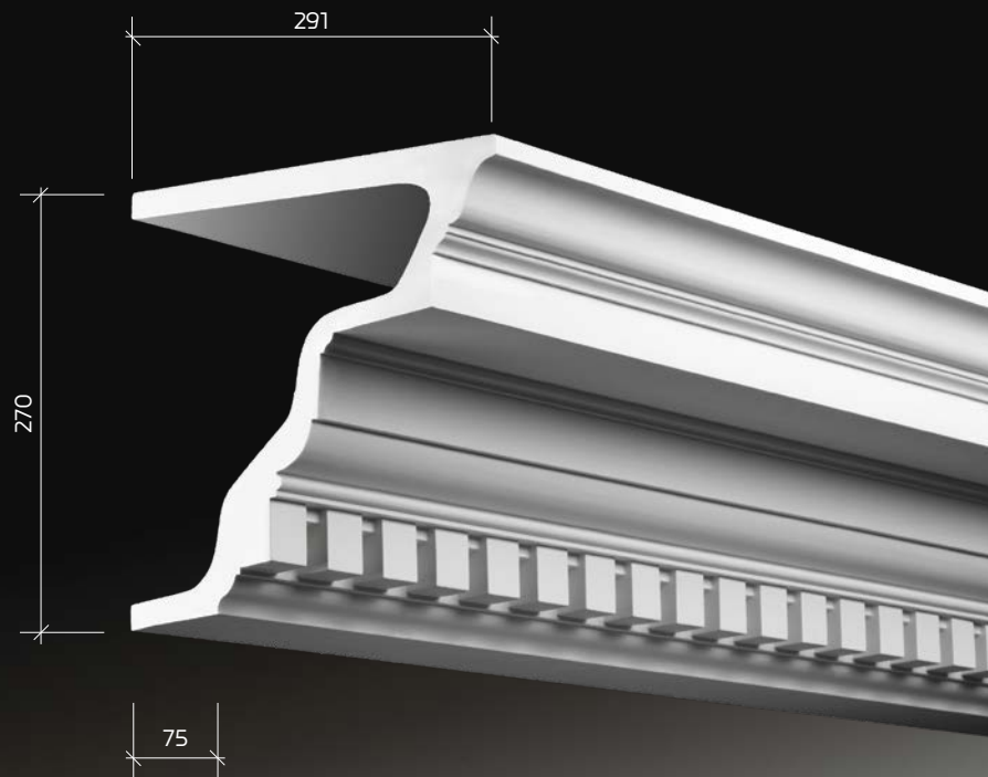
4.02.301 карниз
