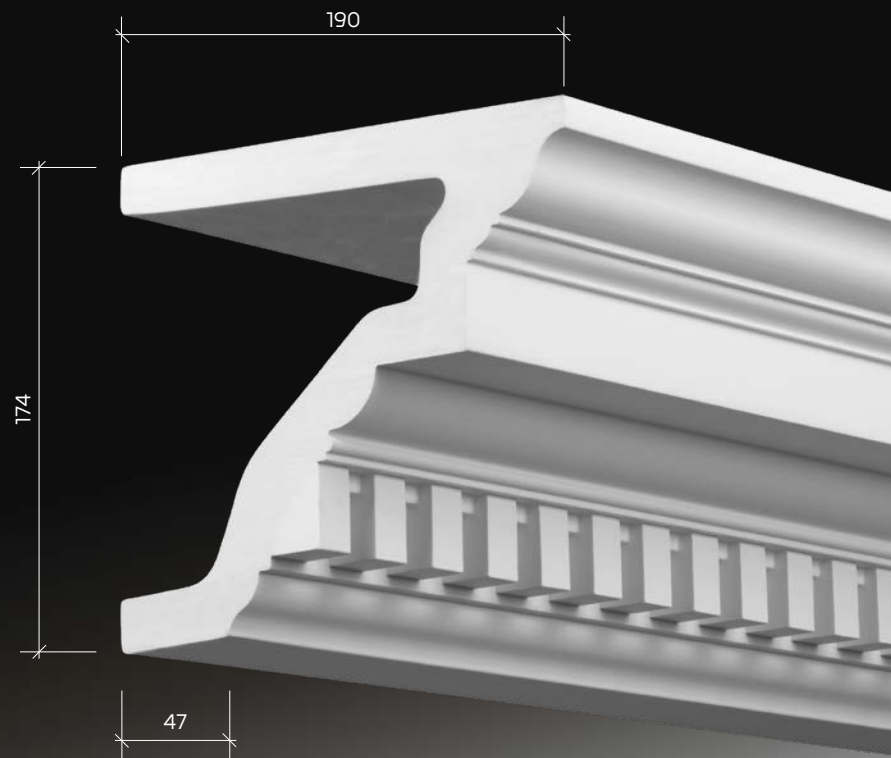
4.32.202 карниз
